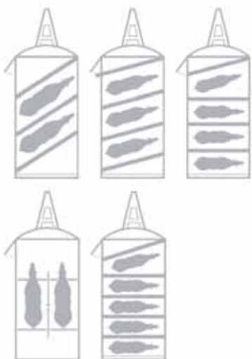
Dispositions typiques des bat-flancs dans le Diagonal 4
